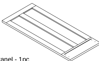
Top Panel - 1pc Panneau supérieur - 1 pièce
